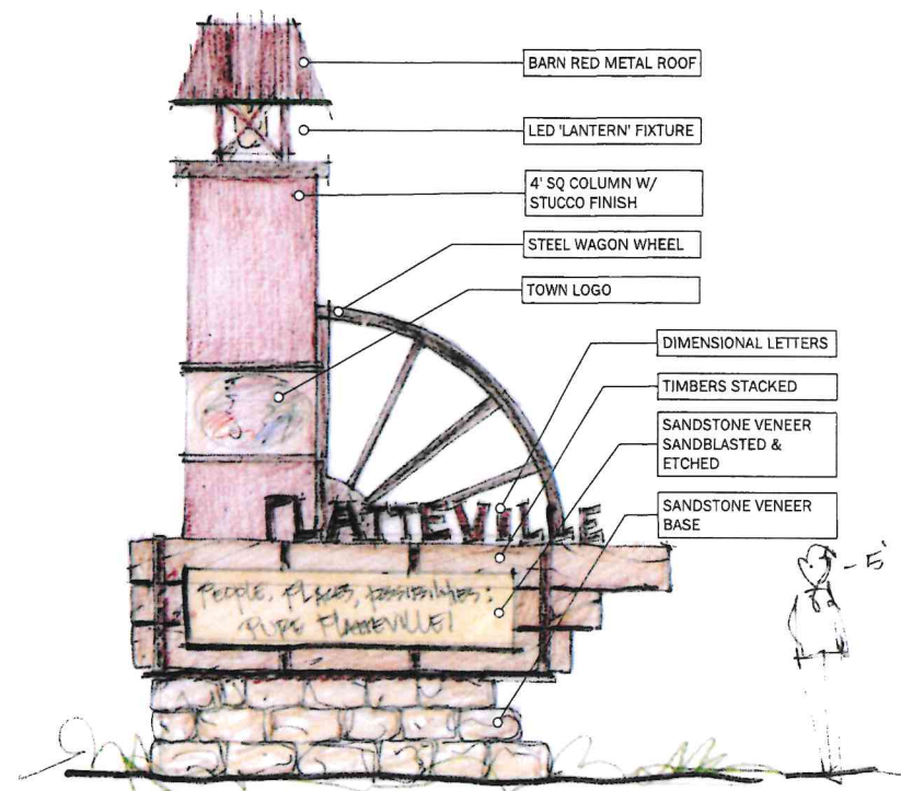
ELEVATION
